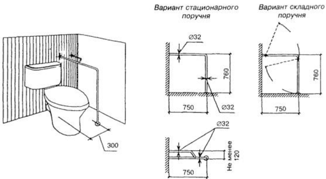
г — устройство двухопорного поручня при унитазе
