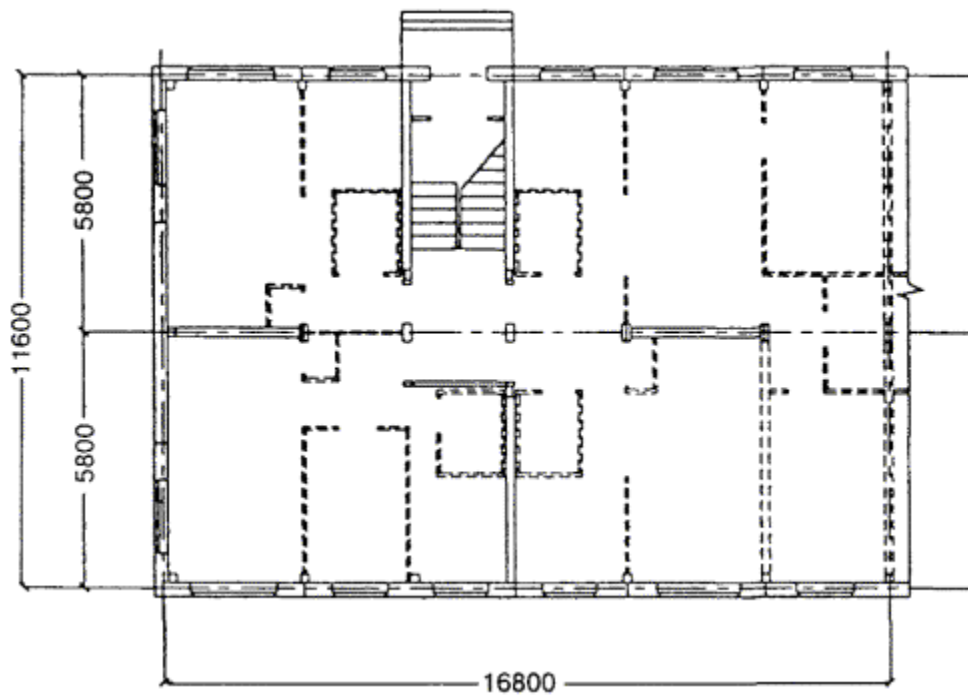
СХЕМА ОРГАНИЗАЦИИ БЛОКА ОБСЛУЖИВАНИЯ В СЕКЦИИ СОЦИАЛЬНОГО ЖИЛЬЯ
