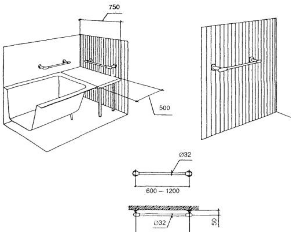
д — схема настенных поручней при ванне
